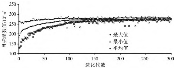
图 5 目标函数值随进化代数变化(方案二)
